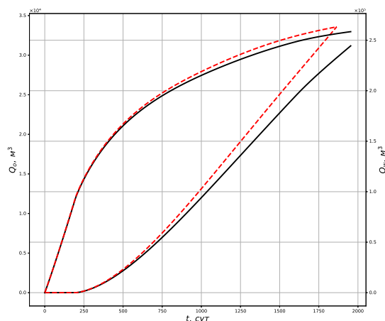
Рис. 2. Накопленные дебиты воды и нефти добывающей скважины
