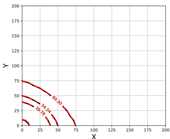
Рис. 3. Поле температуры в момент времени t = 188 суток
