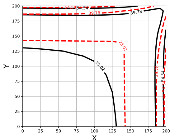
Рис. 4. Поле температуры в момент времени t = 1835 суток
