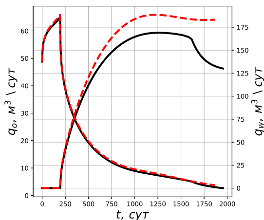
Рис. 1. Дебиты воды и нефти добывающей скважины
